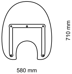
4 PUNTOS DE SUJECIÓN
