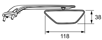
DIMENSIONES (118 x 38 mm)
