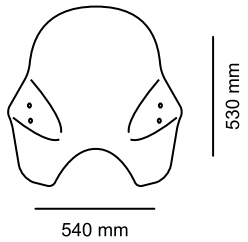
2 PUNTOS DE SUJECIÓN
